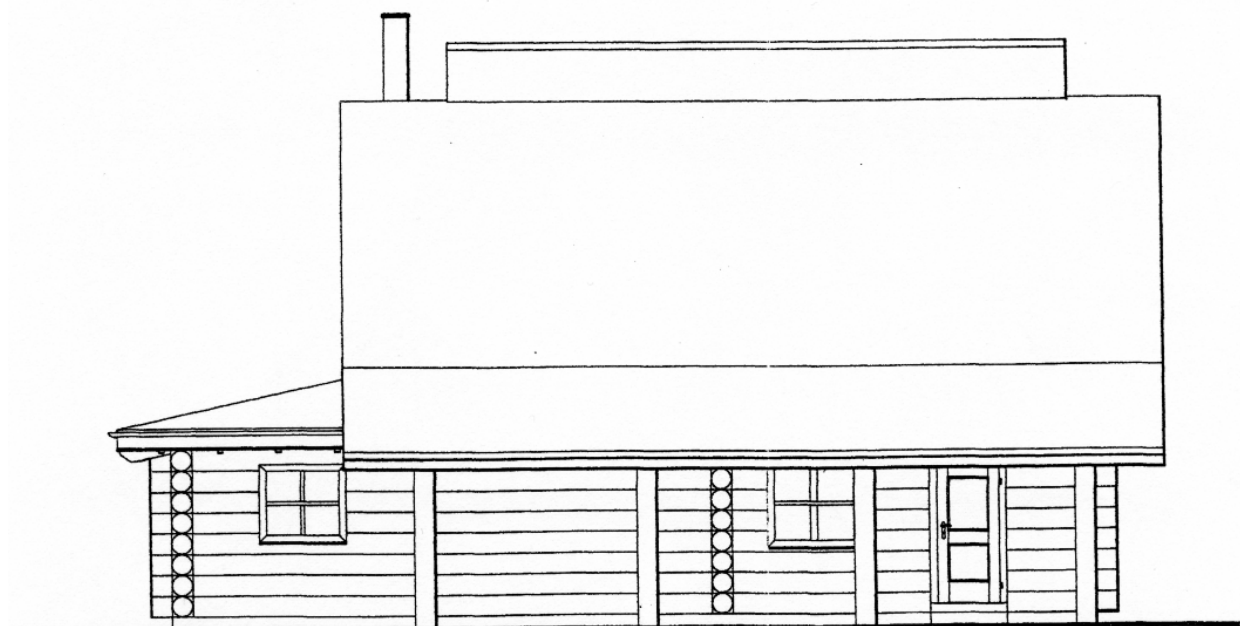
Ansicht Nord
