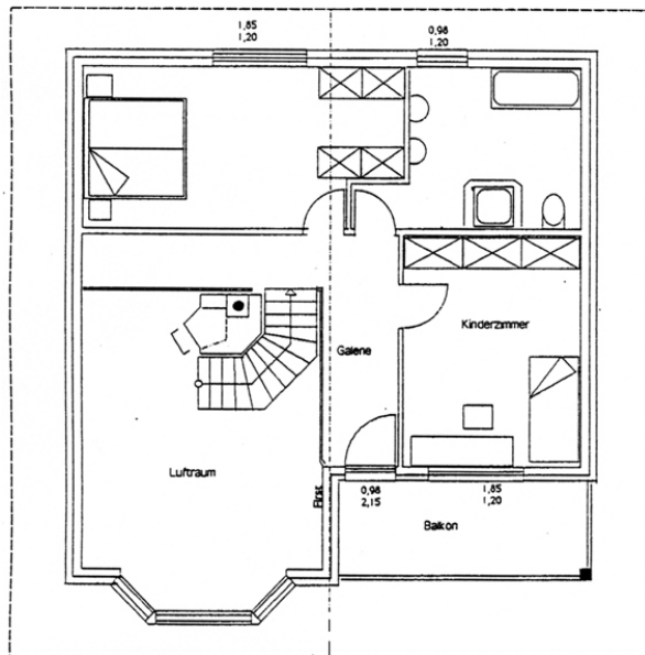
Obergeschoß
