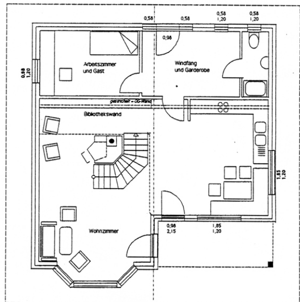
Erdgeschoß
